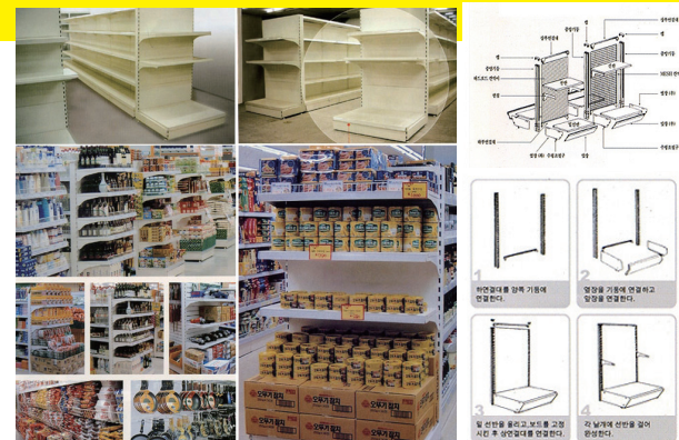
▲ 곤도라용 점볼 BOX(상단용)- 350x900x250 (Stopper, Divider는 별도)
